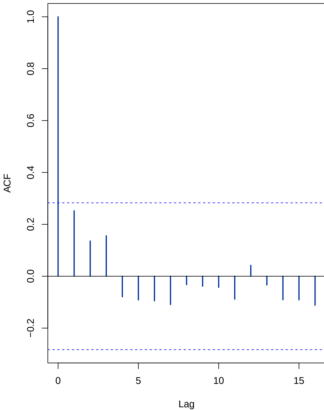
ACF sur résidus OLS ( x \sim t )
