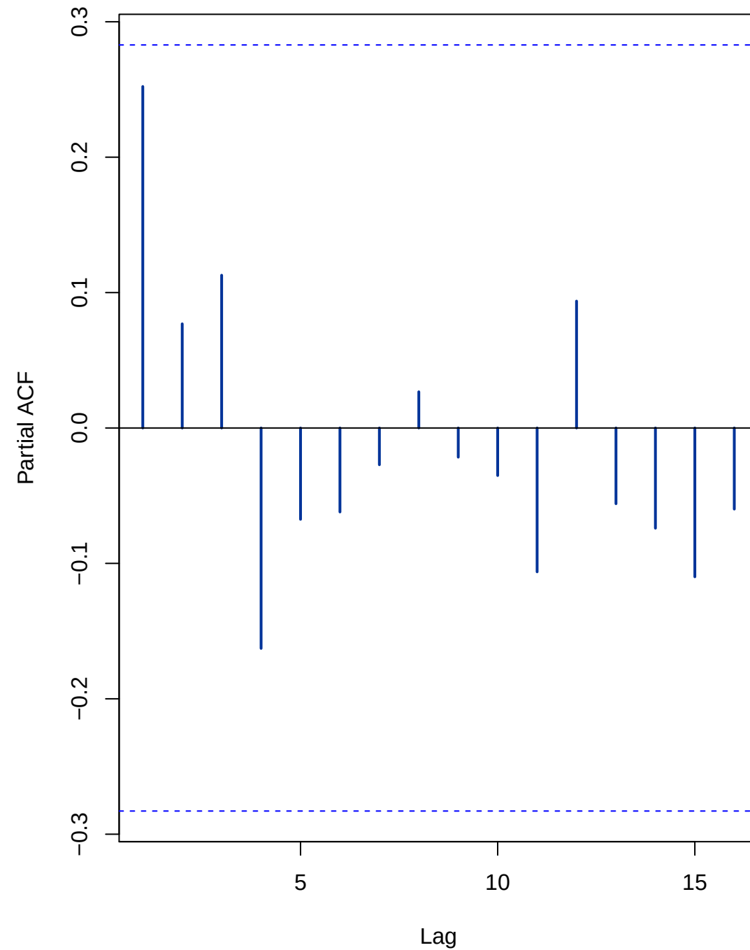
PACF sur résidus OLS ( x \sim t )
